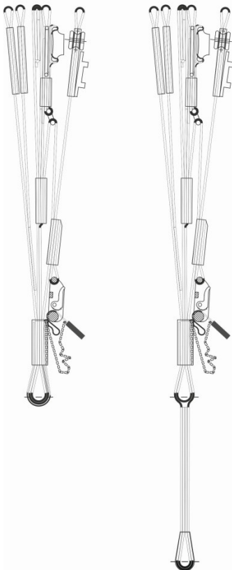
Fig. 3 TWIN RS 2 riser
