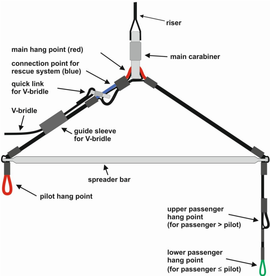
Fig. 8 Tandem spreader bar
